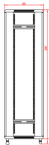
SIDE DOOR
